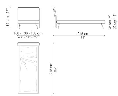
Tonight air Width: 108-138-158cm Depth: 218cm Height: 95cm
