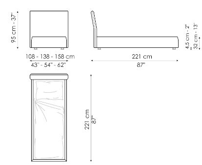
Tonight Width: 108-138-158cm Depth: 221cm Height: 95cm
